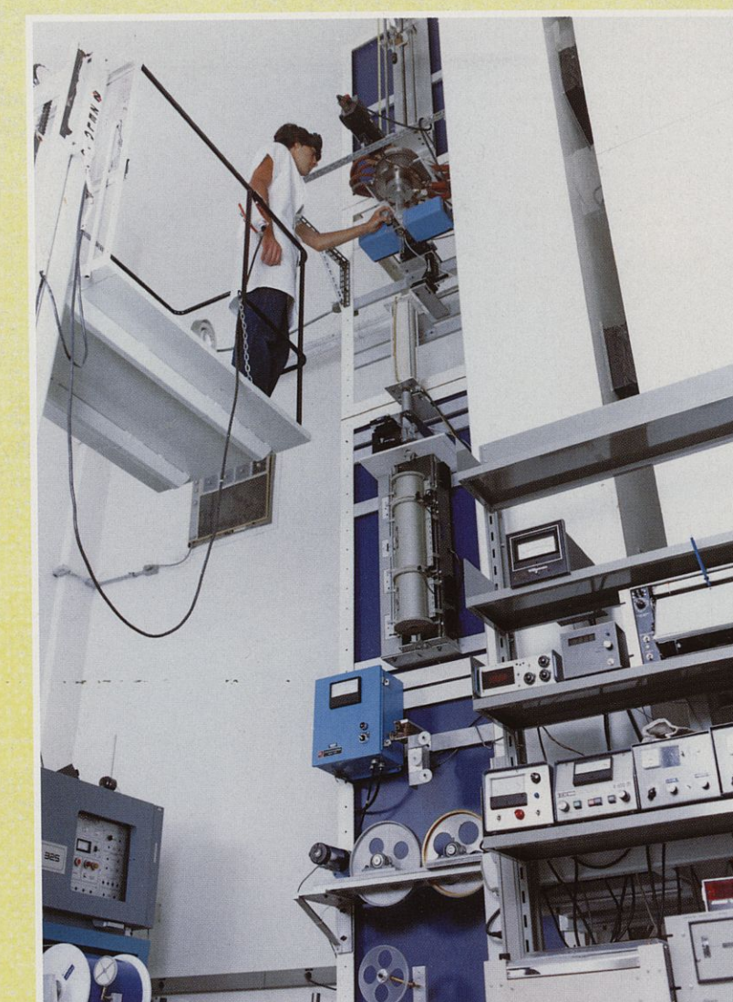
Tirage des fibres optiques au Centre de recherche et développement de TELEBRAS à Campinas (Brésil) (TELEBRAS) Optical fibres pulling at the TELEBRAS Research and Development Centre, Campinas (Brazil) (TELEBRAS) Tracción de fibras ópticas en el Centro de Investigación y Desarrollo de TELEBRAS en Campinas (Brasil) (TELEBRAS)
